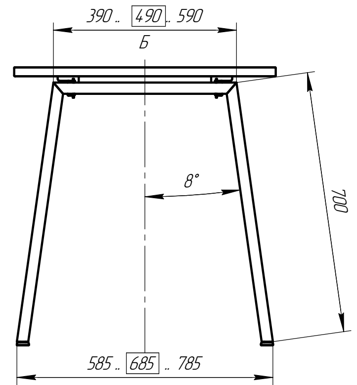
Размеры стандартных элементов прямых столов МК Каппа 60x30 TP
