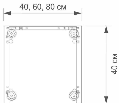
вид сверху
